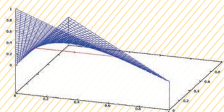
統計学で有名な「シンプソンのパラドックス」を情報幾何を使って表現したもの
